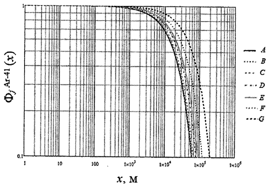
Рис. 3. Графики зависимостей функции истощения для ^{41}\text{Ag} от расстояния от источника для различных категорий устойчивости атмосферы
